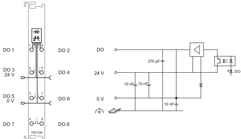
Abb. 2.1.1-3: 8-Kanal Digital Ausgangsklemme 750-530
