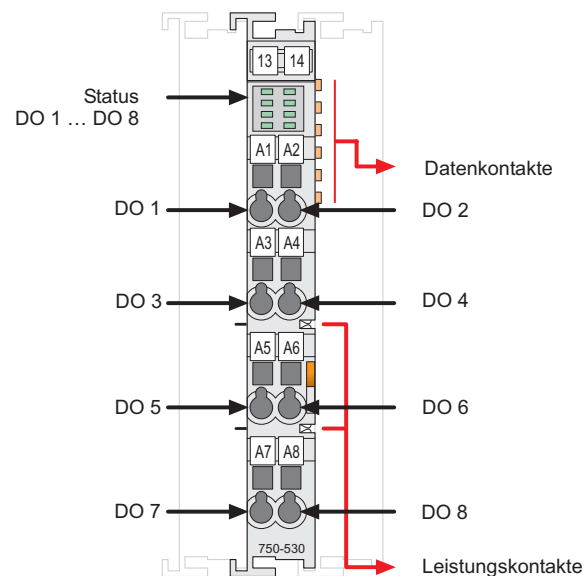
Abb. 2.1.1-1: 8-Kanal Digital Ausgangsklemme 750-530
